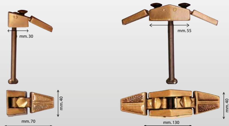
Art. 30954 Perno da Ø 8 MA x 90 compreso nel prezzo
