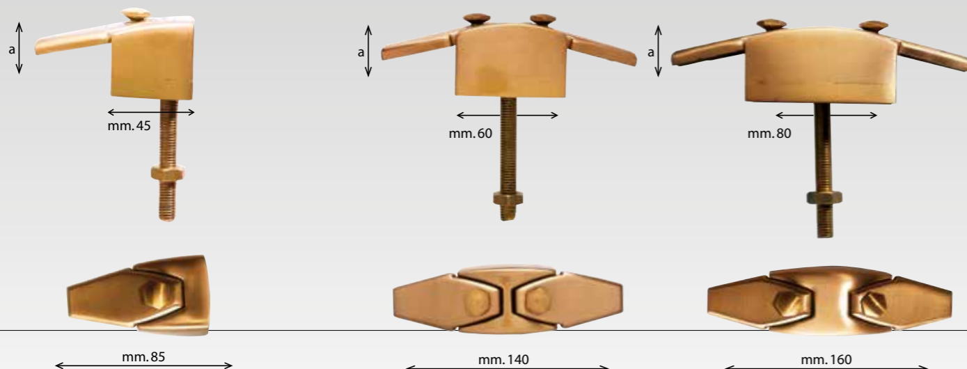
Art. 30770 - a = cm. 2-3 Perno da Ø 10 MA x 100 compreso nel prezzo Art. 30773 - a = cm. 2-3 Perno da Ø 8 MA x 100 compreso nel prezzo Art. 30771 - a = cm. 2-3 Perno da Ø 10 MA x 100 compreso nel prezzo Art. 30774 - a = cm. 2-3 Perno da Ø 8 MA x 100 compreso nel prezzo Art. 30772 - a = cm. 2-3 Perno da Ø 10 MA x 100 compreso nel prezzo Art. 30775 - a = cm. 2-3 Perno da Ø 8 MA x 100 compreso nel prezzo
