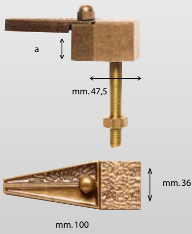
ART. 30952 a = 1 cm. ART. 30950 a = 2 cm. Perno da Ø 10 MA x 100 compreso nel prezzo
