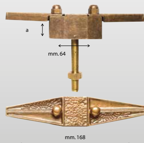
ART. 30953 a = 1 cm. ART. 30951 a = 2 cm. Perno da Ø 10 MA x 100 compreso nel prezzo
