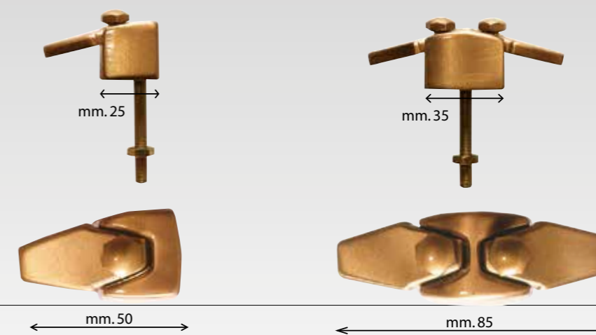
Art. 30977 Perno da Ø 8 MA x 100 compreso nel prezzo Art. 30978 Perno da Ø 8 MA x 100 compreso nel prezzo
