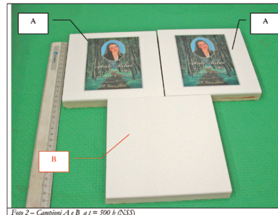
Foto 2 - Campioni A e B a t = 500 h (NSS)
